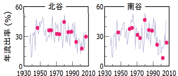
図 竜ノ口山森林理水試験地において実測された流出率（ \sim ）の経過と流域平均林冠高から推定した流出率（ \bullet ）の分布
